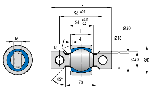
Fig. 5 Spherical Mount 054 18 710, 054 18 711
