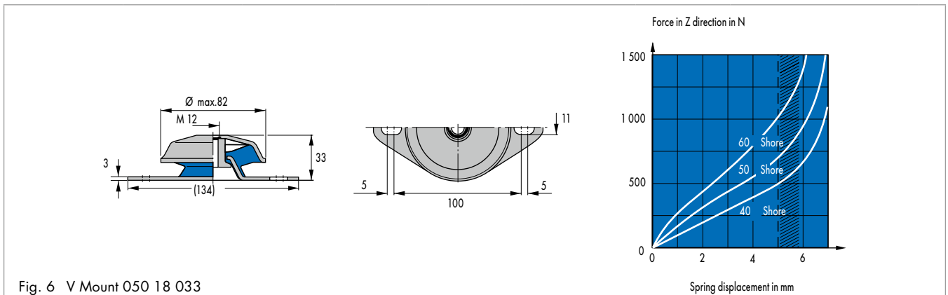
Fig. 6 V Mount 050 18 033
