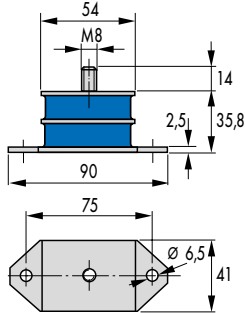
Fig. 3 Flat Mount 051 18 001
