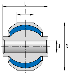
Fig. 3 Spherical Mounts 054 18 036, 054 18 068, 054 18 191, 054 18 070
