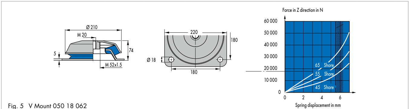
Fig. 5 V Mount 050 18 062
