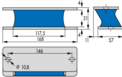
Fig. 4 Flat Mount 051 18 004
